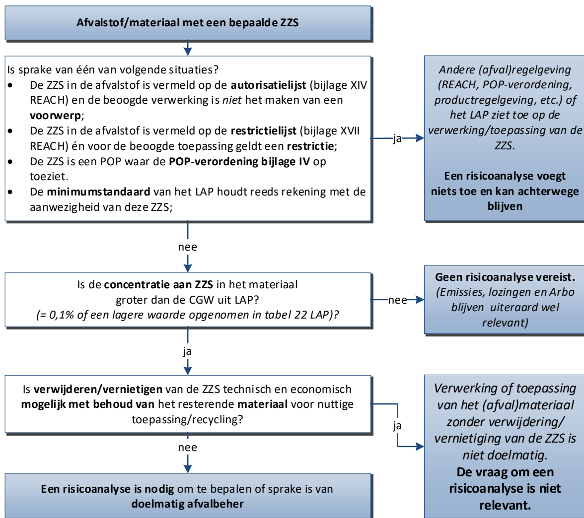
figuur 2 Schematische weergave van situaties waarin de risicoanalyse wordt uitgevoerd
